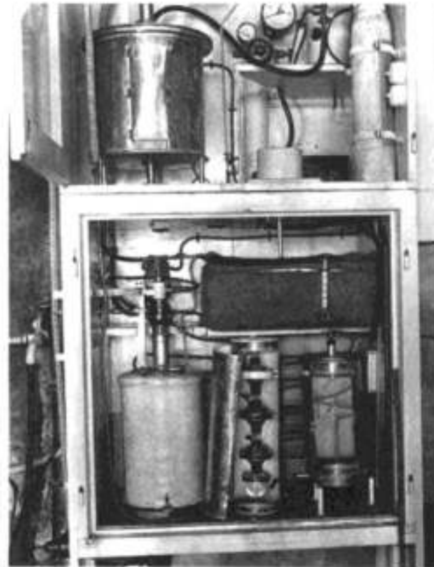
Apparatur zur Herstellung quellwasserähnlichen Trinkwassers.
